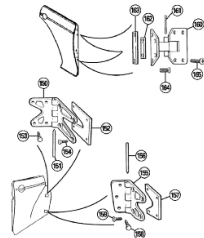
Hinges
